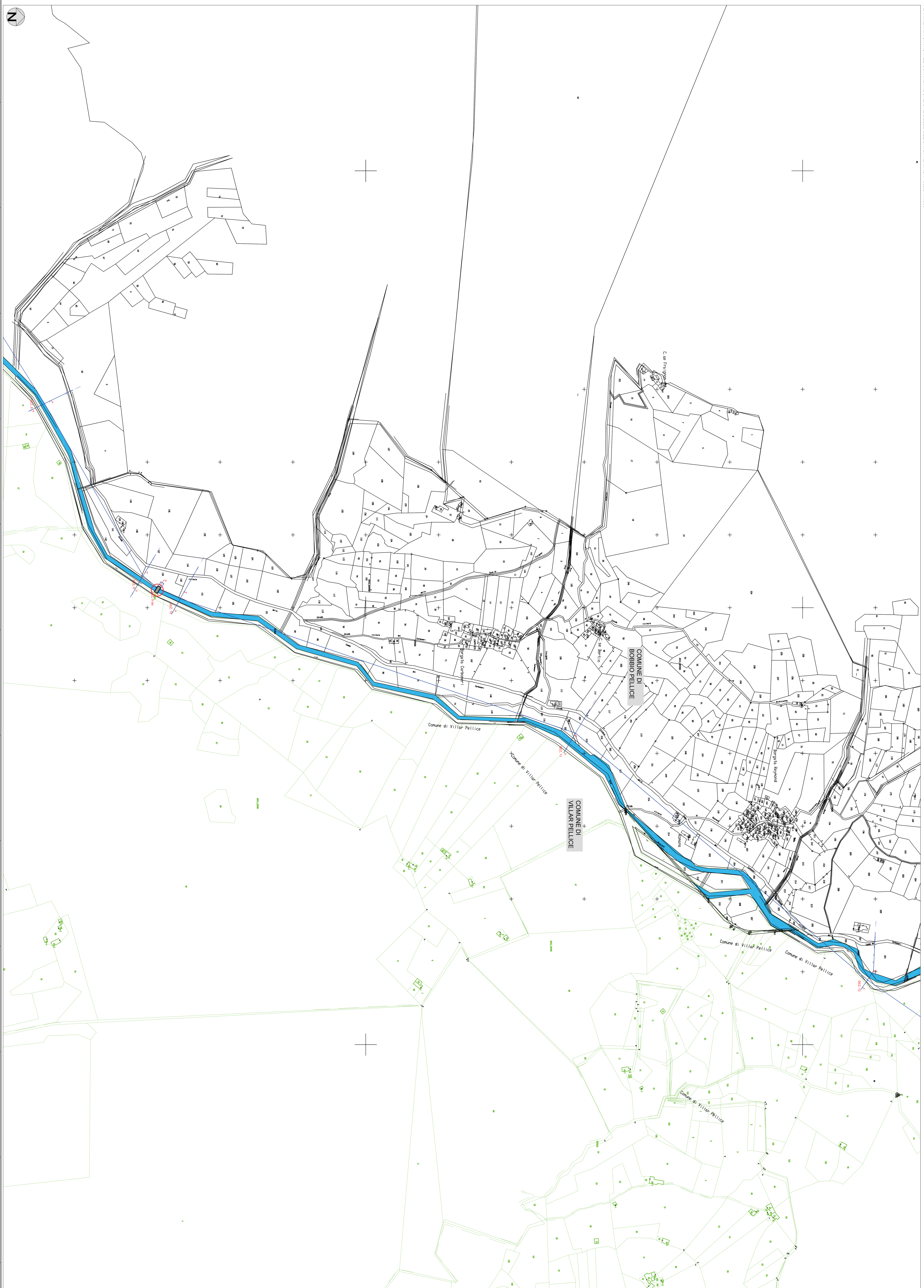
PLANIMETRIA CATASTALE CON INDICAZIONE DELLE SEZIONI DI VERIFICA - scala 1:1500
