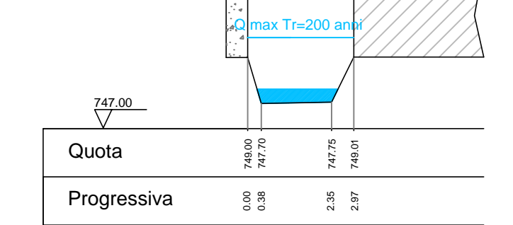
Sez. 3
