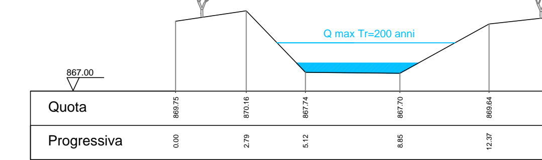
Sez. 10
