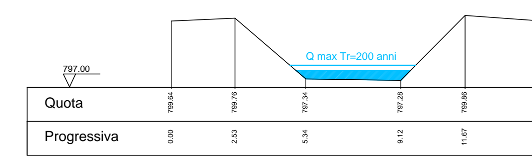
Sez. 6
