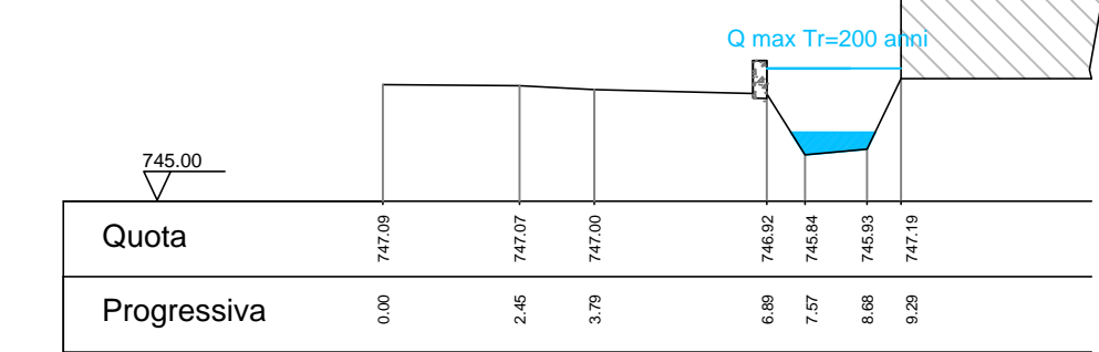
Sez. 2
