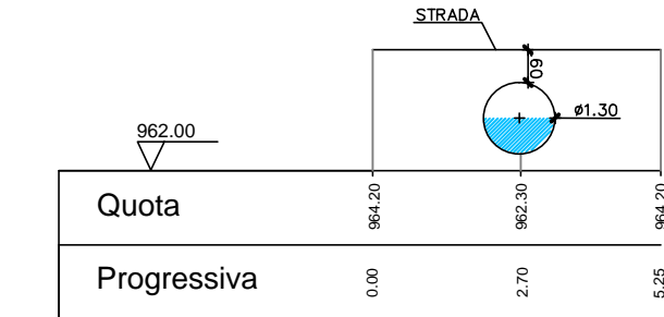
Attraversamento P6
