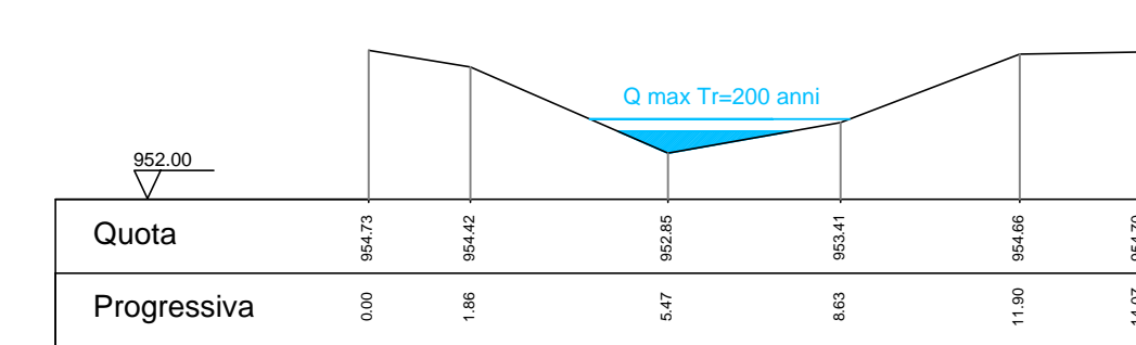
Sez. 14
