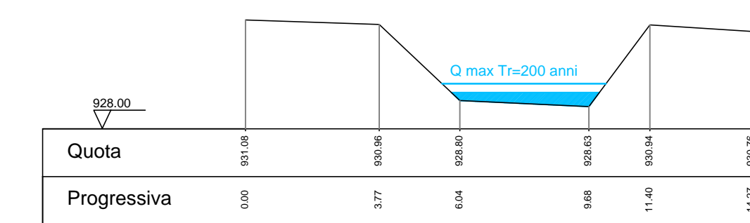
Sez. 13
