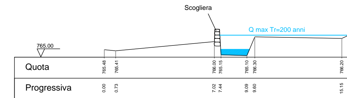
Sez. 4
