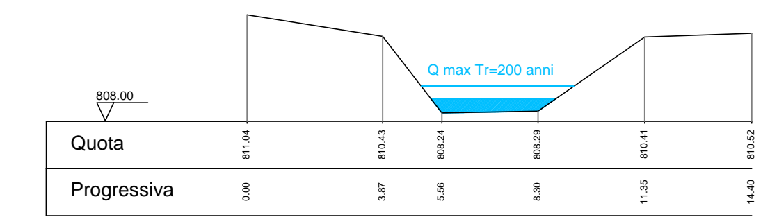
Sez. 7
