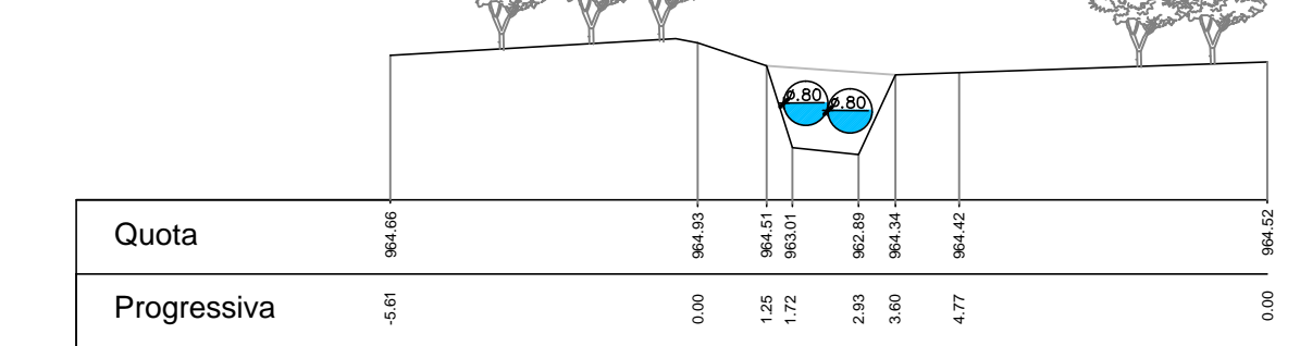
Attraversamento P7
