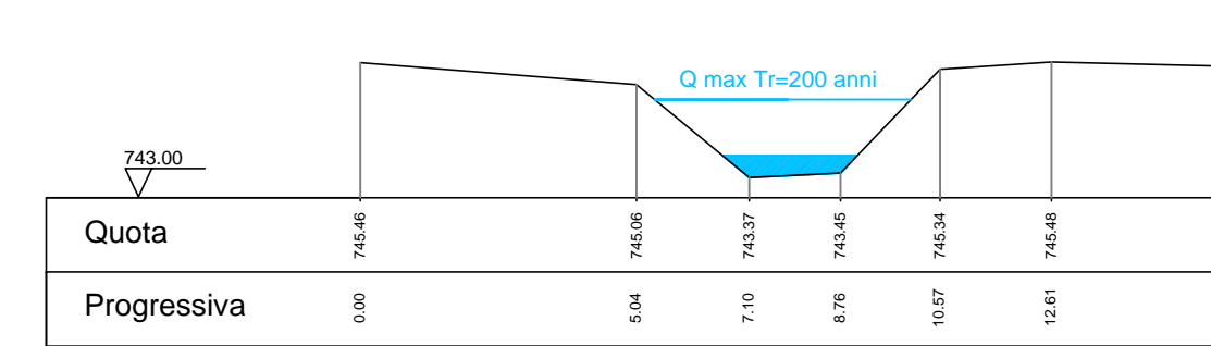
Sez. 1
