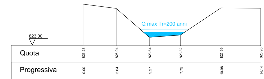
Sez. 8
