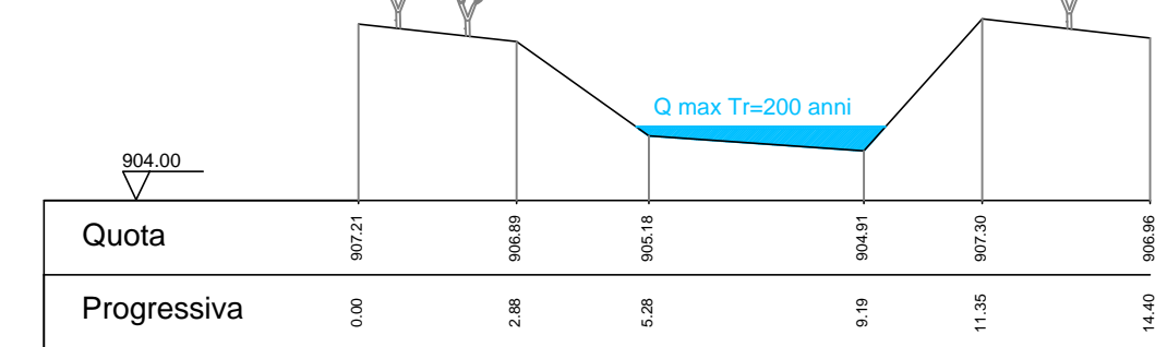
Sez. 12
