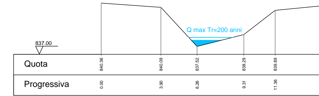
Sez. 9
