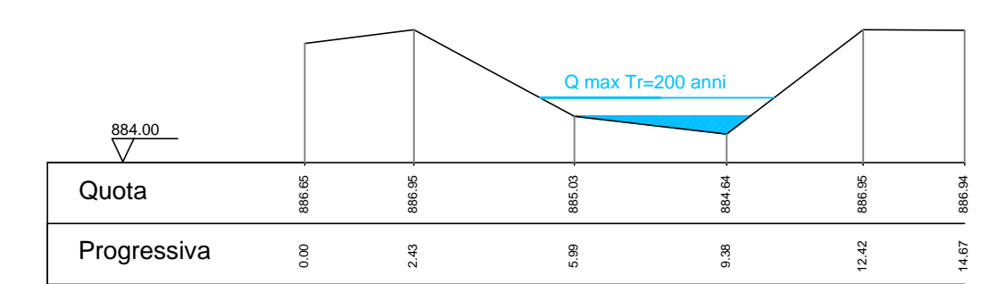
Sez. 11
